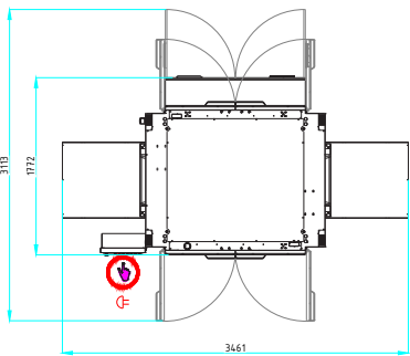
Altura de la máquina 2730 mm
