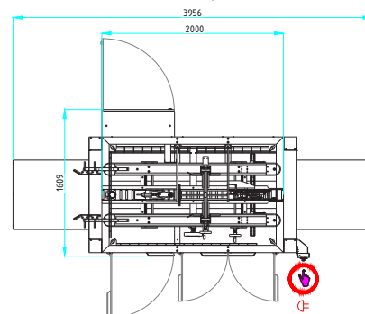
Altura máquina: 2385 mm
