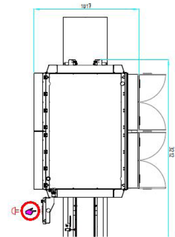
Maschinenhöhe bei geschlossener Folienrollentür: 2095 mm Maschinenhöhe bei geöffneter Folienrollentür: 2255 mm
