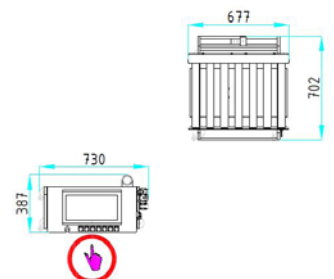
Kontrollwaage mit Bedienfeld
