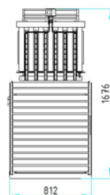
Kontrollwaage mit Ausschleusung
