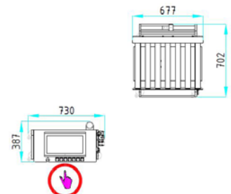
Trieuse pondérale avec panneau de commande
