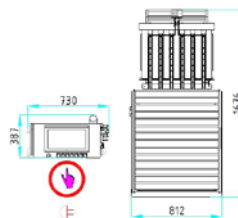
Trieuse pondérale, rejet et panneau de commande
